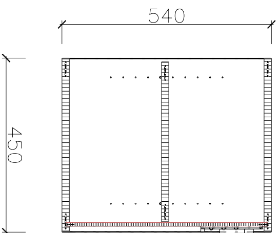
Schnitt G-G
